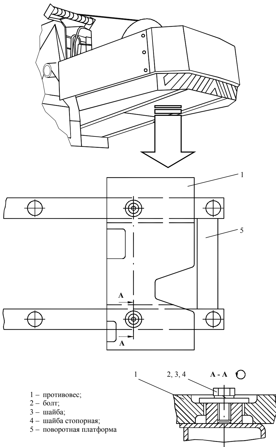
Рисунок 3.1 – Установка противовеса
