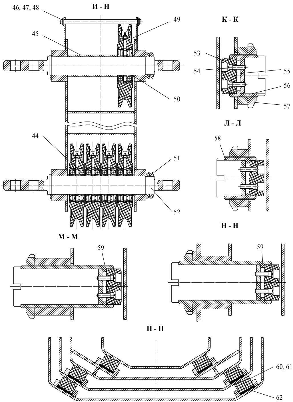
Рисунок 3.17.4 - Стрела телескопическая
