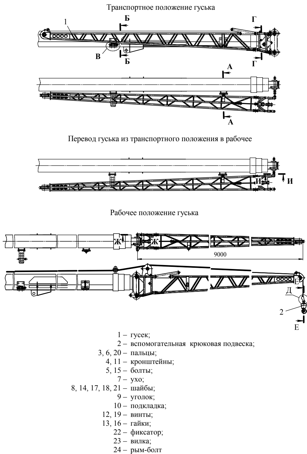
Рисунок 3.20.1 – Сменное стреловое оборудование
