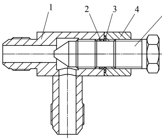
Дроссель ДР6
