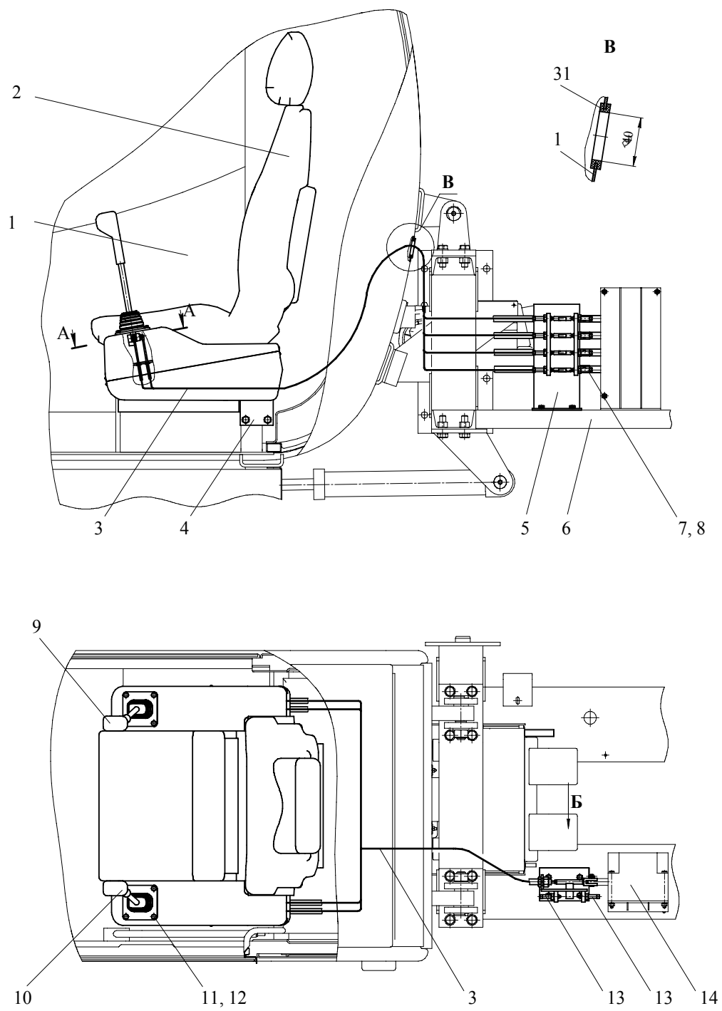
Рисунок 3.22 – Схема приводов
