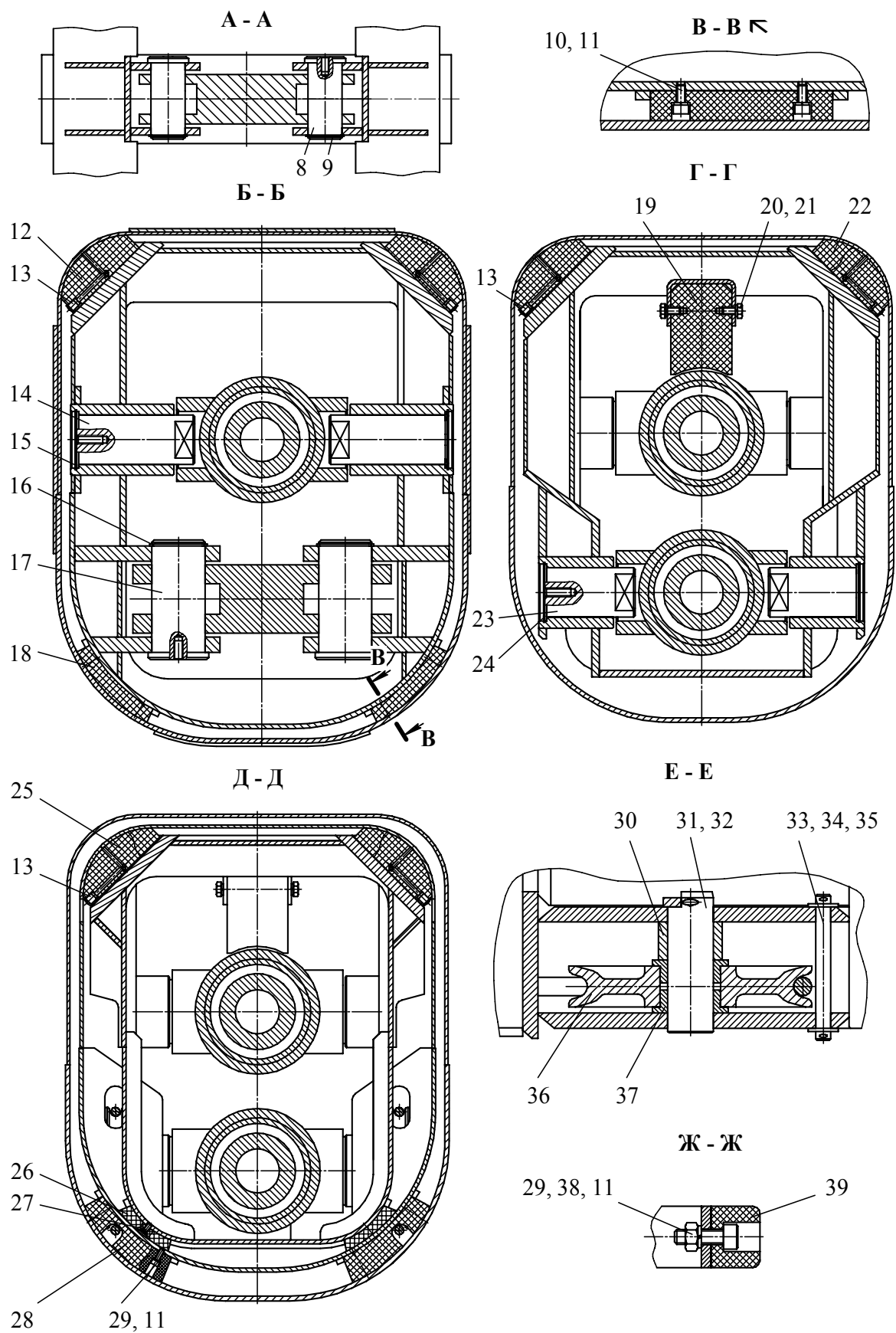
Рисунок 3.17.2 – Стрела телескопическая
