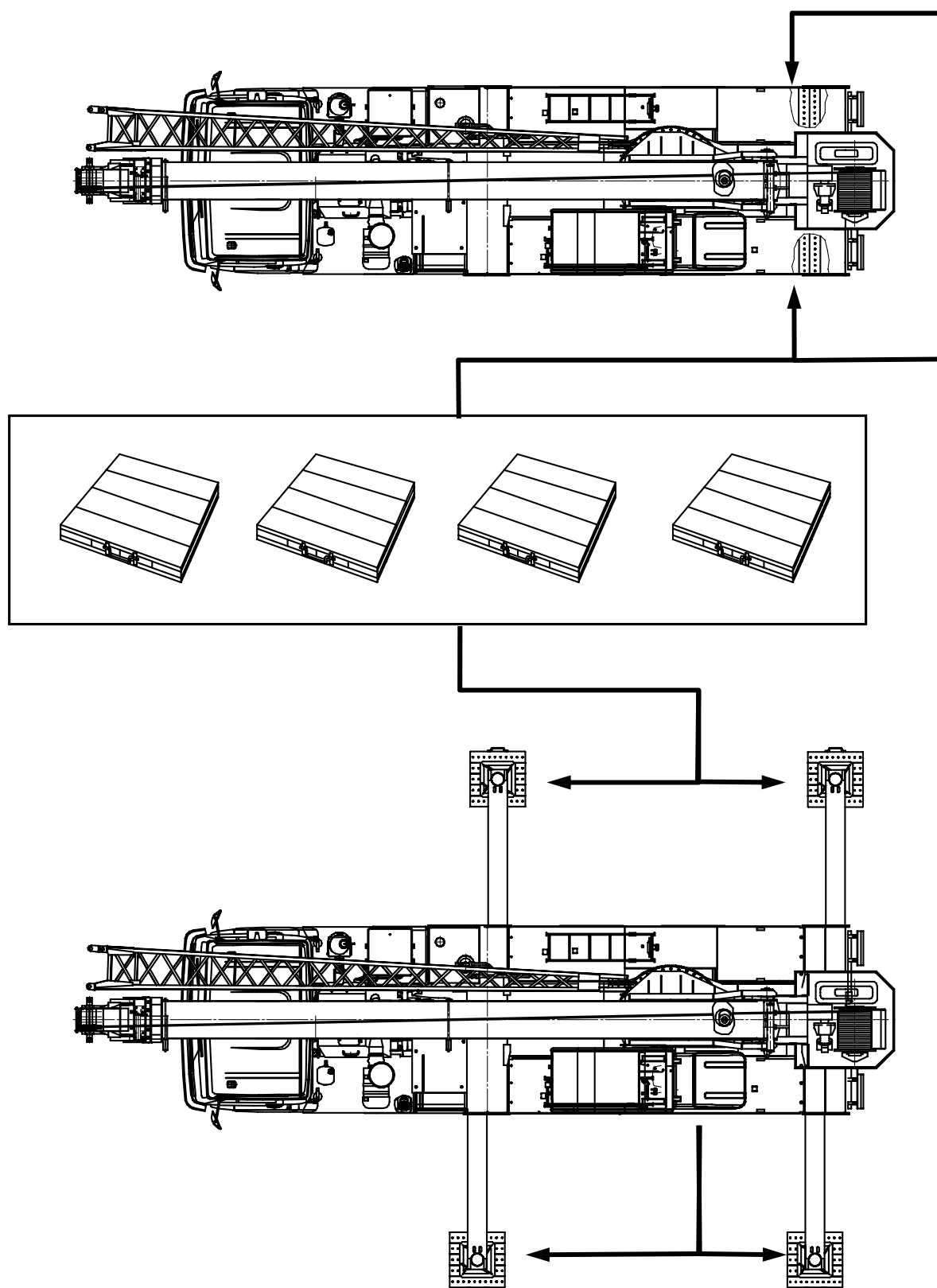
Рисунок 2.9 – Размещение инвентарных подкладок в транспортном и рабочем положениях крана
