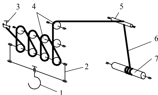
Схема четырехкратной запасовки грузового каната
