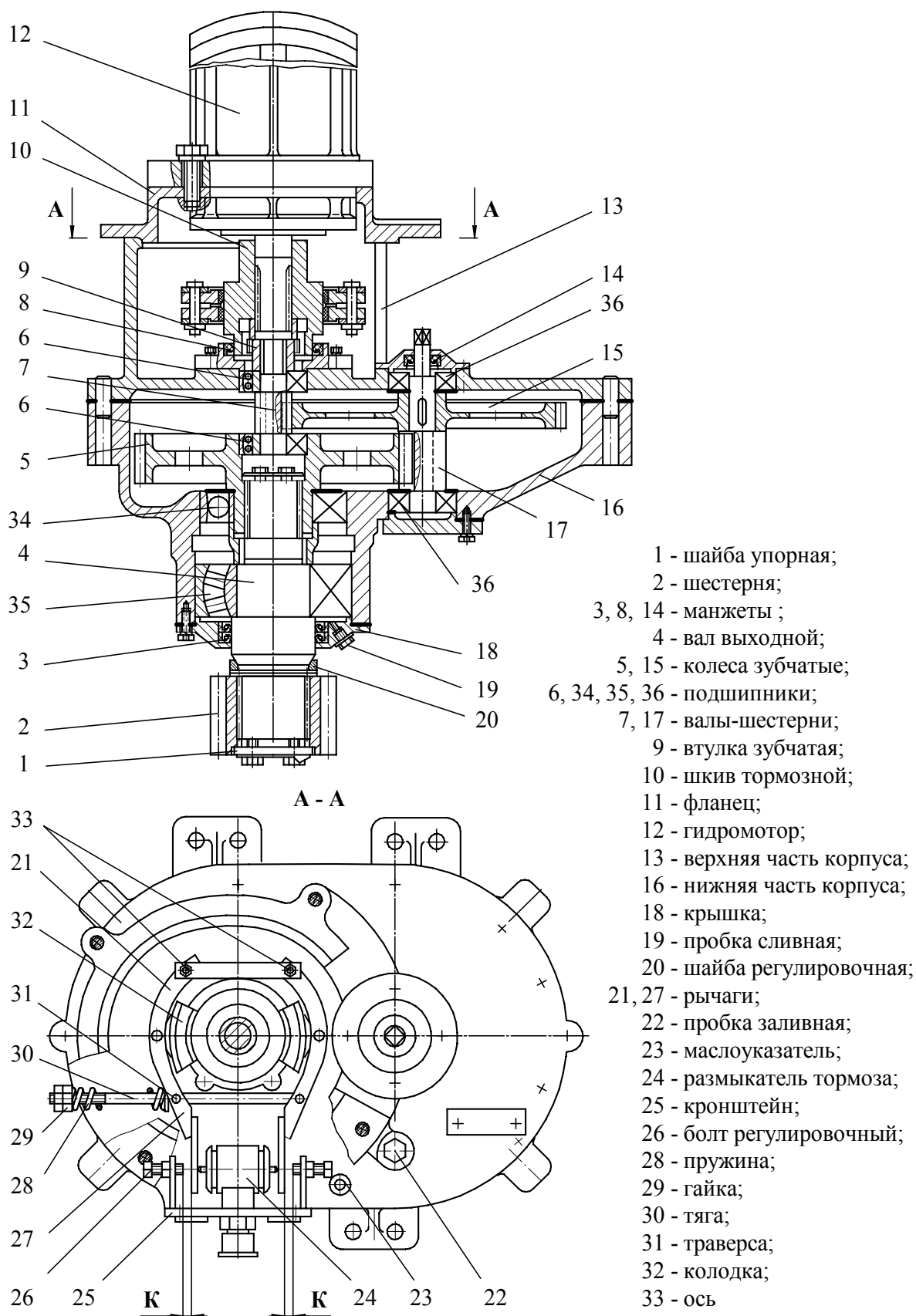
Рисунок 3.9 – Механизм поворота
