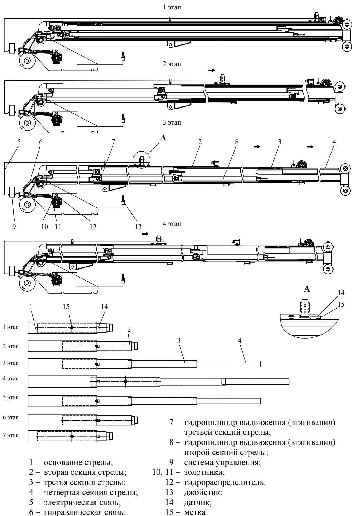
Рисунок 3.18 – Схема телескопирования стрелы
