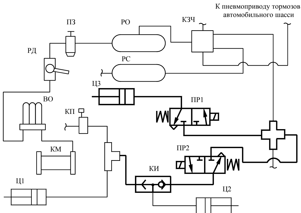
Рисунок 3.23 – Схема пневматическая принципиальная
