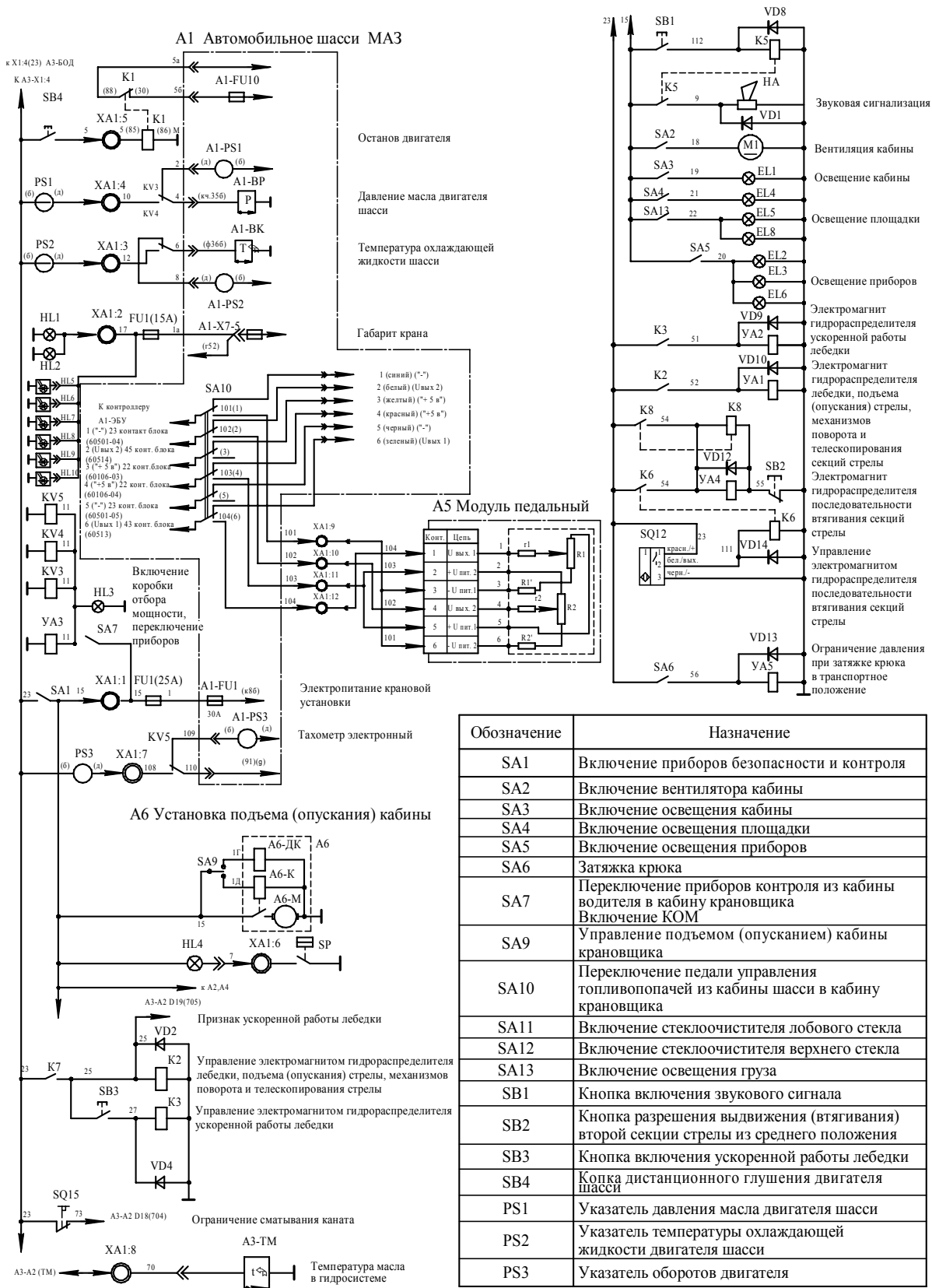
Рисунок 5.1 – Схема
