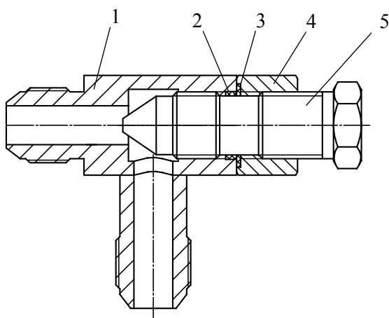
Дроссель ДР6
