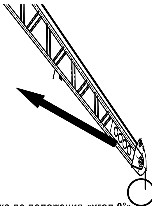
Рисунок 13.29 – Подъем гуська до положения «угол 0°»
