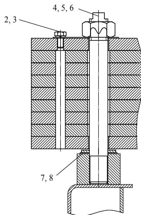
Рисунок 3.1 – Установка противовеса
