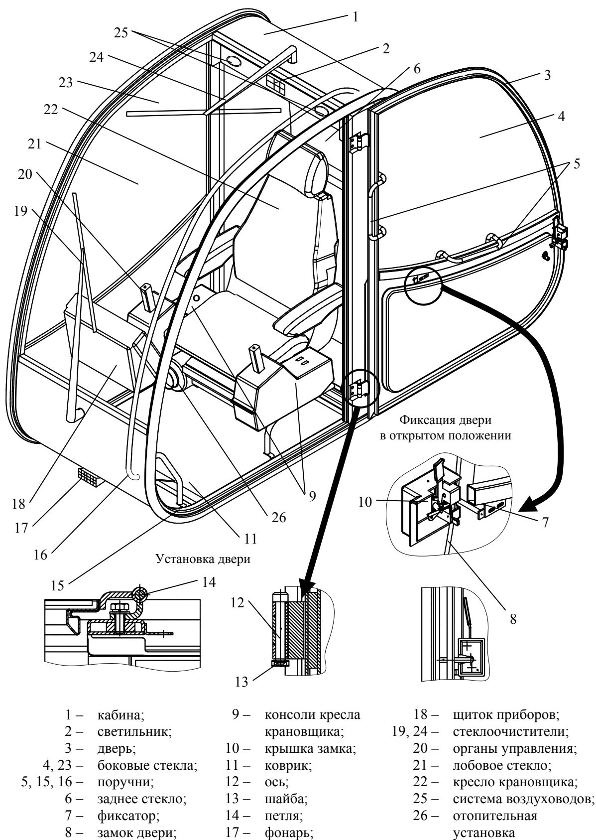
Рисунок 3.4 – Устройство кабины крановщика
