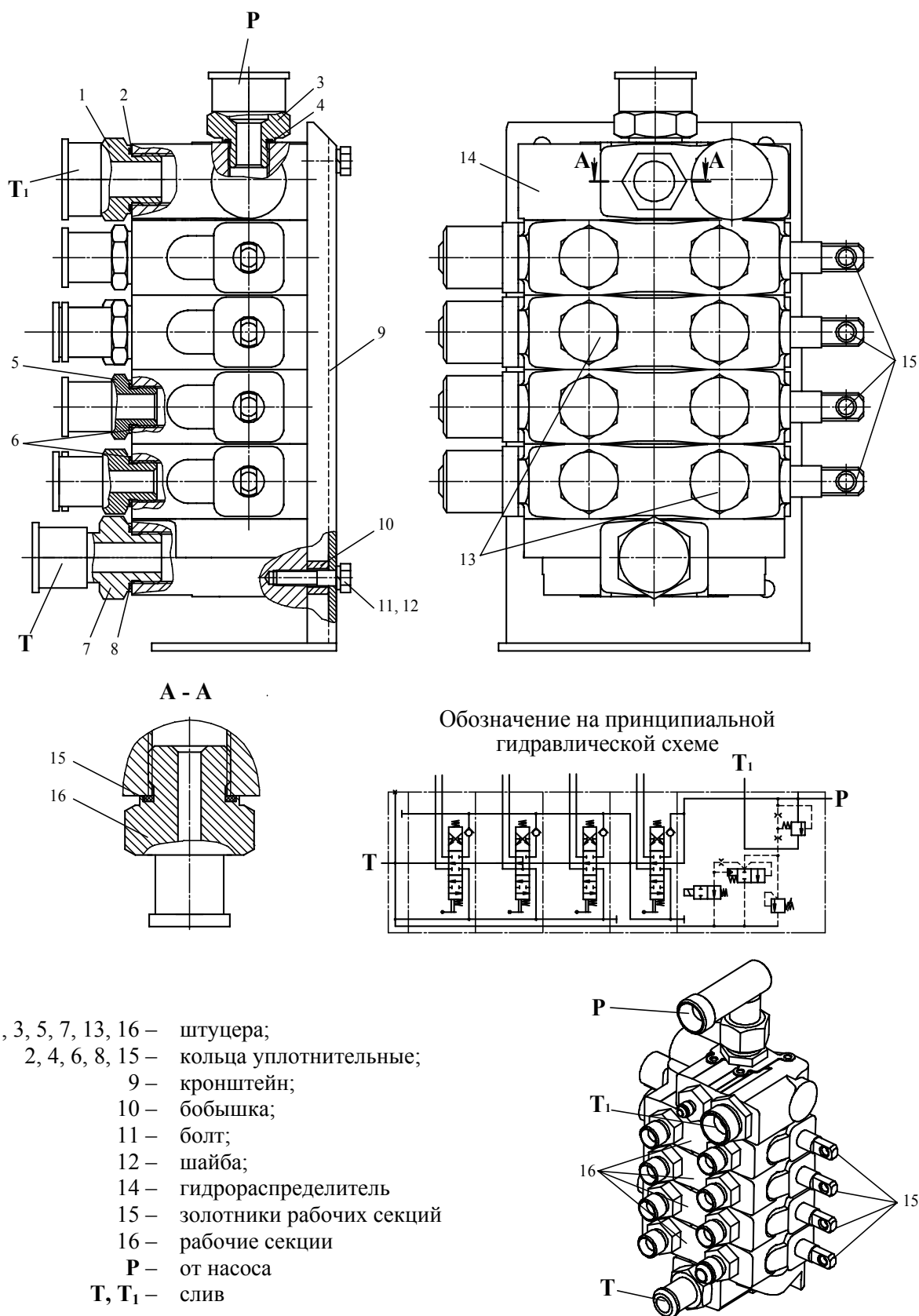
Рисунок 4.6 – Гидрораспределитель управления крановыми операциями
