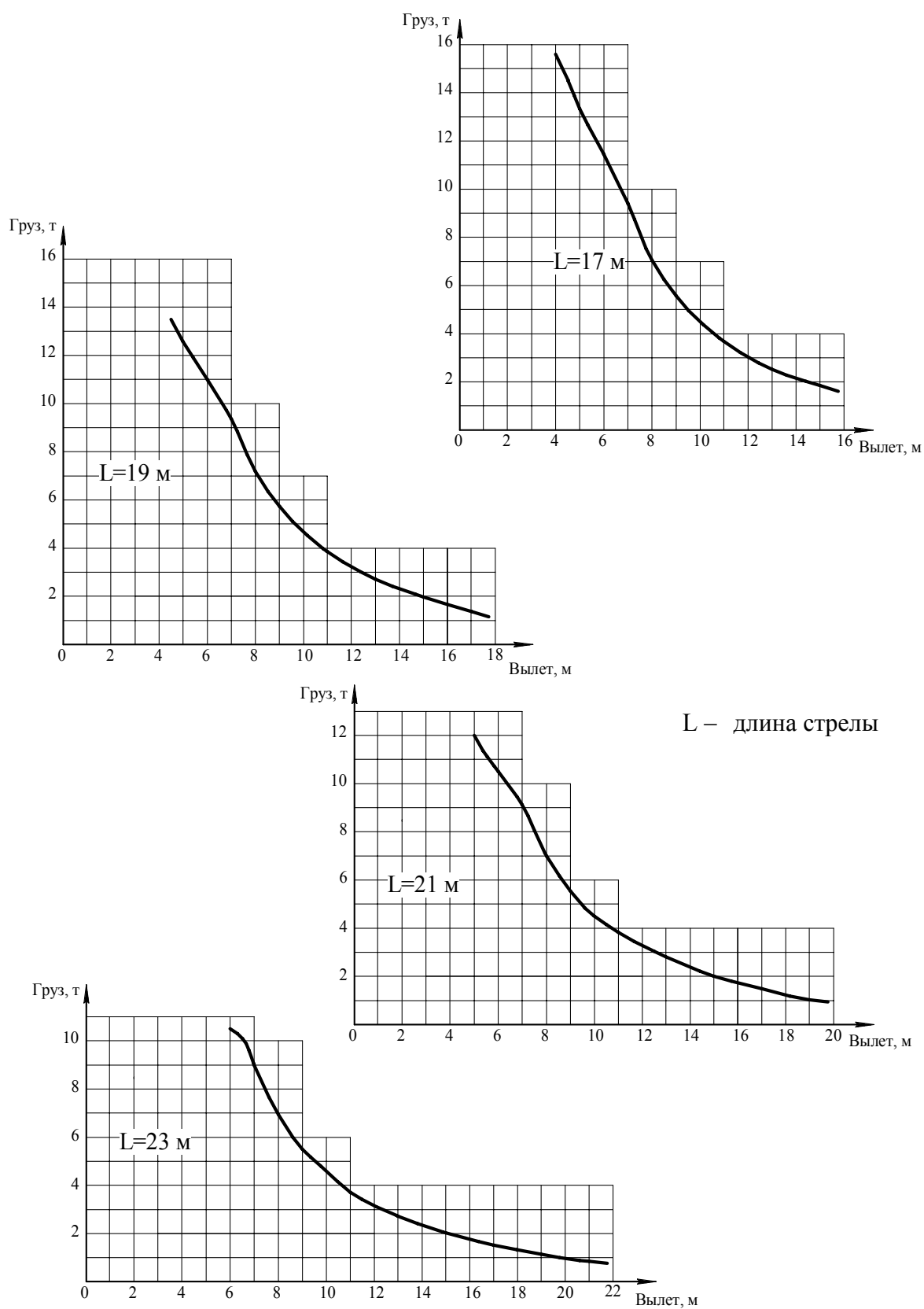
Рисунок А.2.2 – Грузовые характеристики крана на выдвинутых выносных опорах в зоне работы 360°
