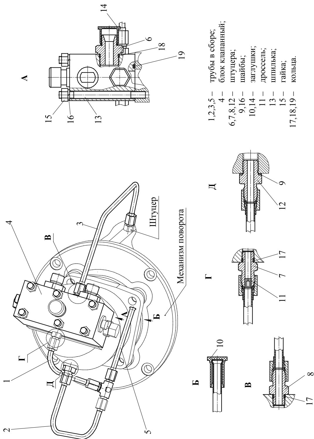
Рисунок 4.32 – Гидрооборудование механизма поворота
