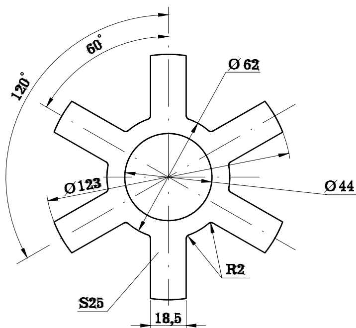
Рисунок К.14 - Звездочка KC-3577.26.032-3
