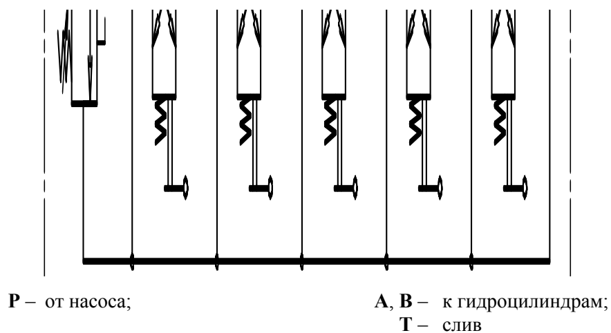
Рисунок 4.5 – Гидрораспределитель управления выносными опорами
