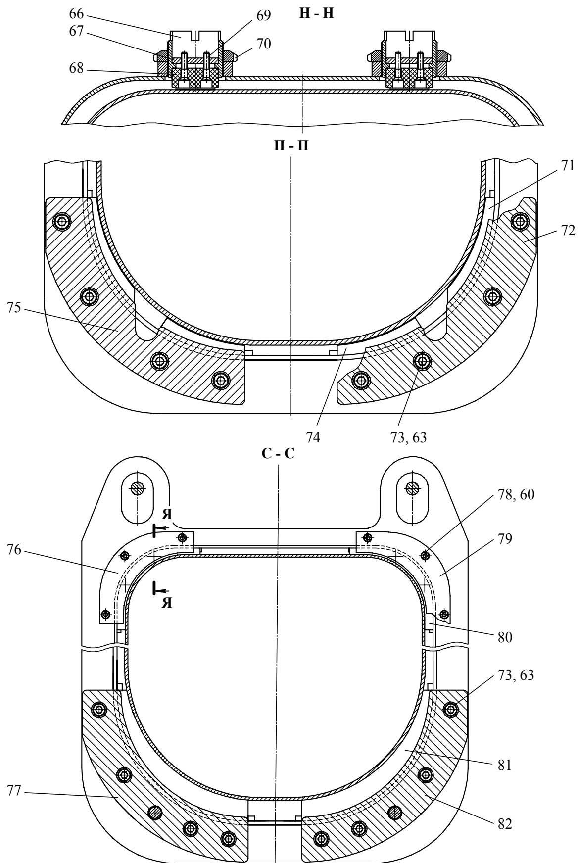
Рисунок 3.17.4 – Стрела телескопическая
