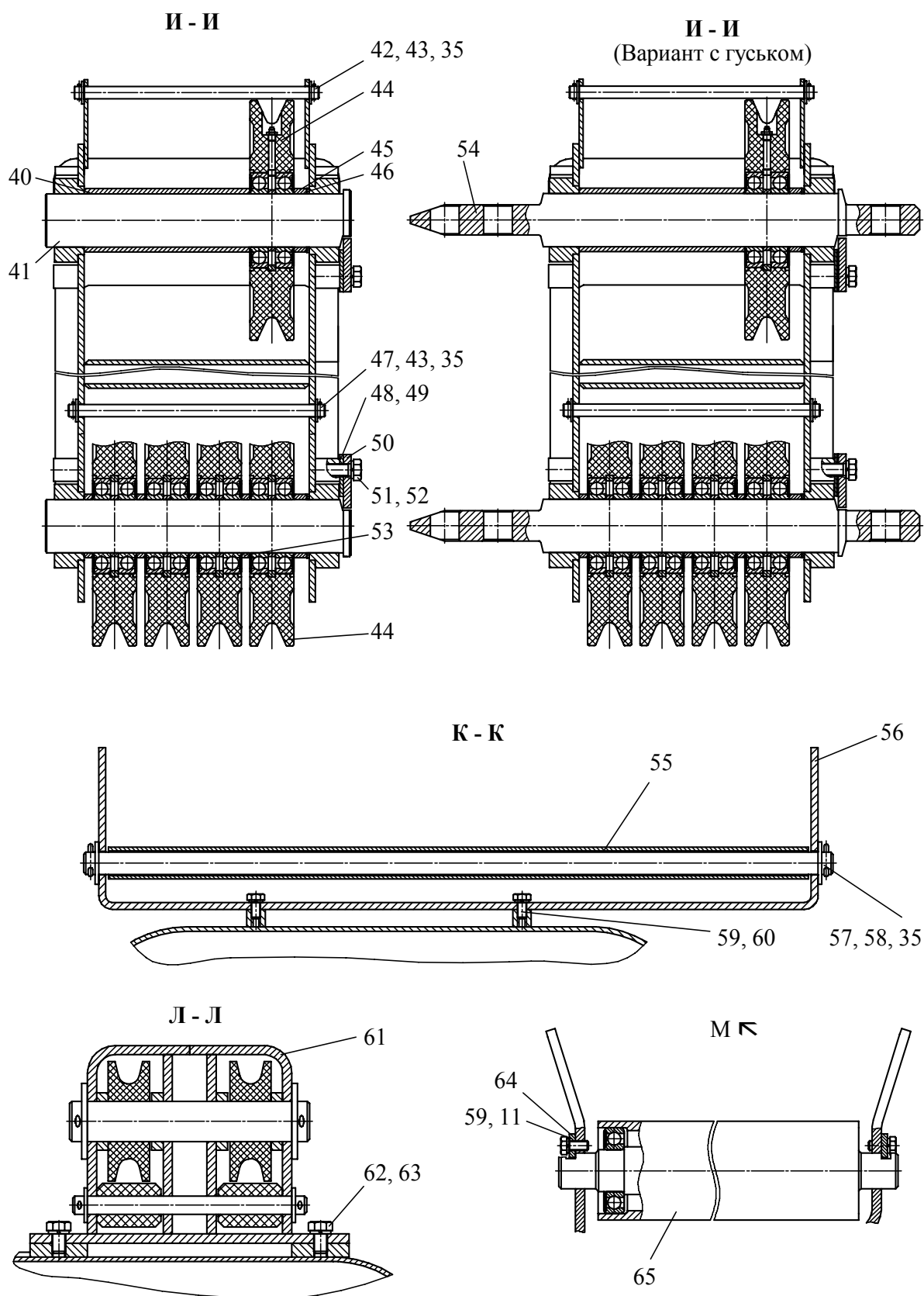
Рисунок 3.17.3 – Стрела телескопическая
