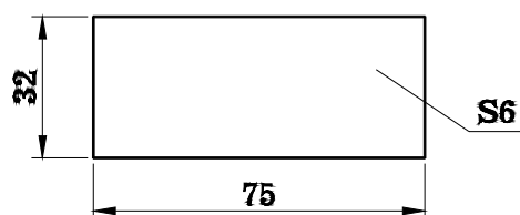
Рисунок К.15 - Лента тормозная KC-3577.28.032
