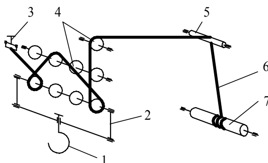
Схема четырехкратной запасовки грузового каната
