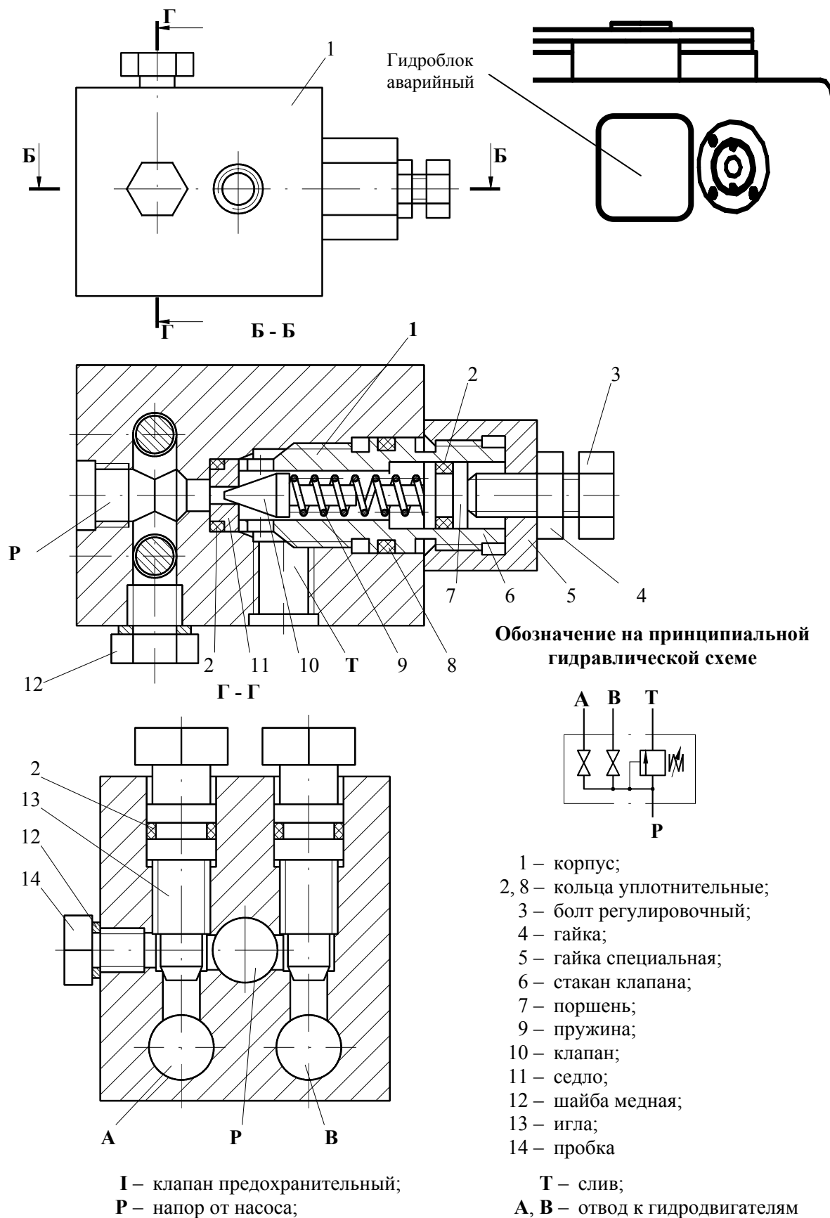
Рисунок 4.25 – Гидроблок аварийный
