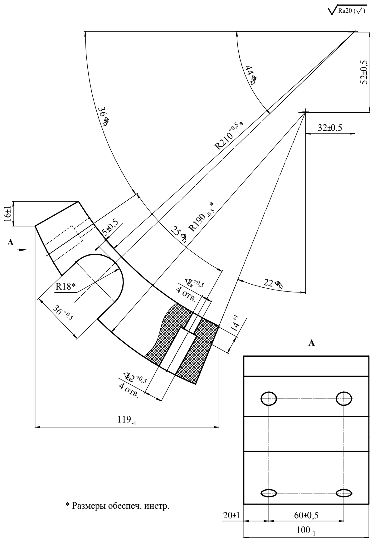
Рисунок К.11 – Опора скольжения задняя нижняя КС-54712.63.112-1
