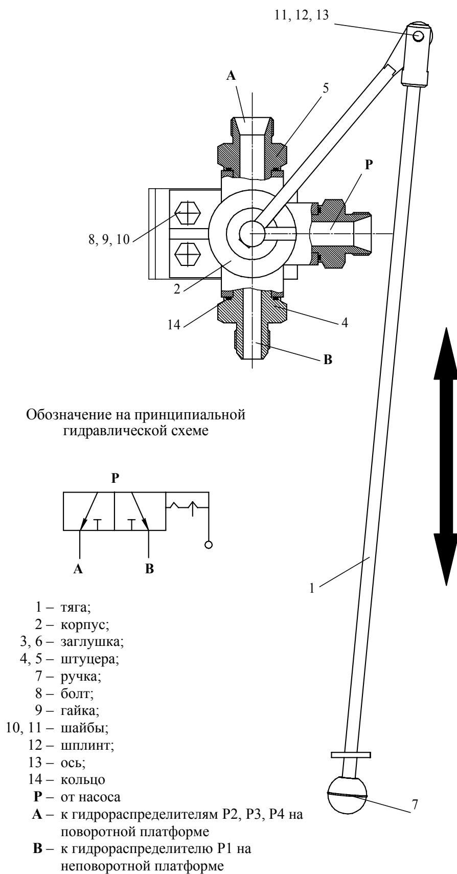
Рисунок 4.26 – Кран трехходовой
