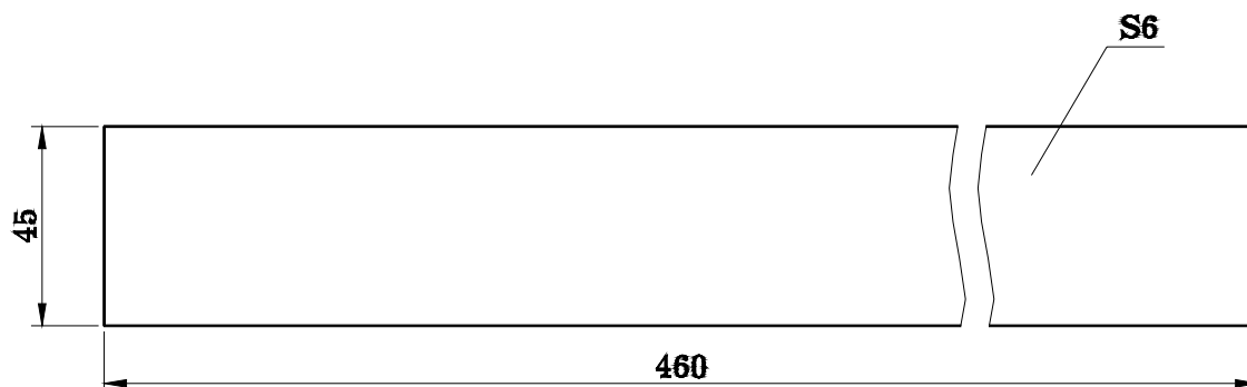
Рисунок К.15 - Лента тормозная KC-3577.28.032
